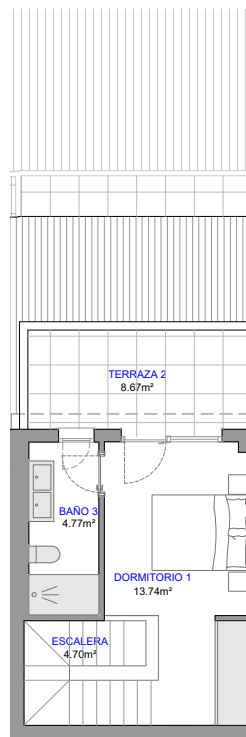
PLANTA SEGUNDA
