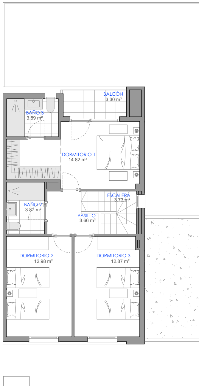
PLANTA PRIMERA
